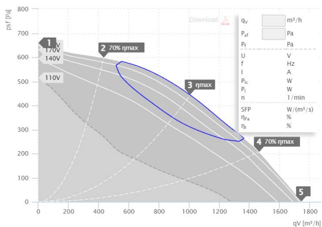
MPC 225 E2 T21 | 137885 (230V)
