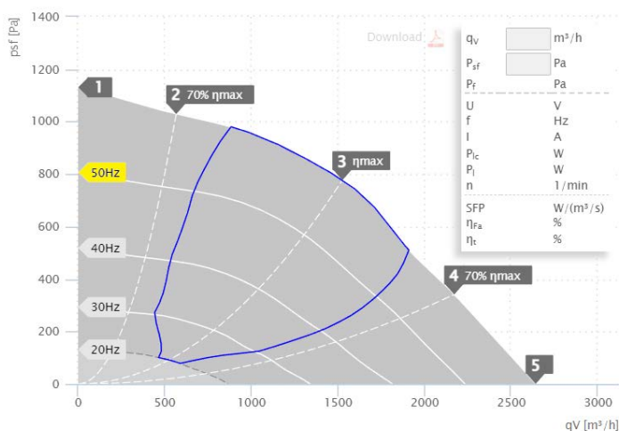
MPC 250 D2 T40 | 157209 (400V)
