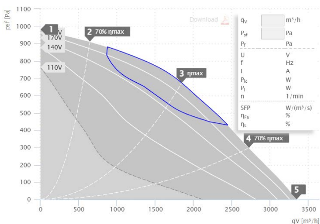
MPC 280 E2 T20 | 126681 (230V)
