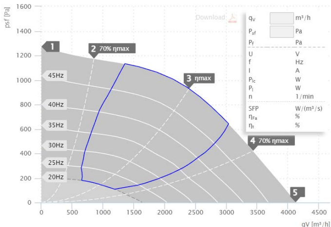
MPC 315 D2 T40 | 157218 (400V)
