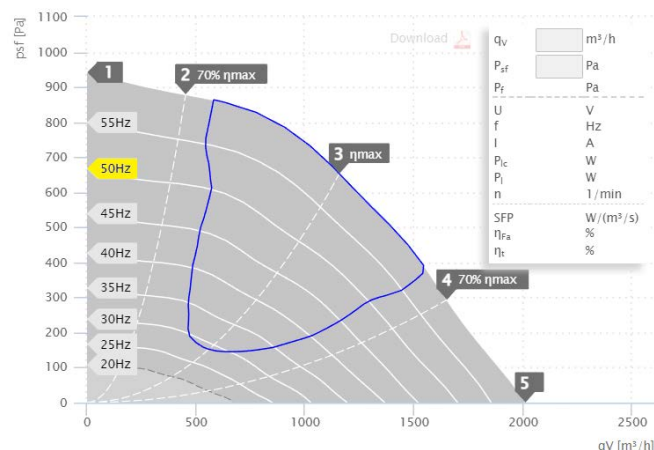
MPC 225 D2 T40 | 157206 (400V)
