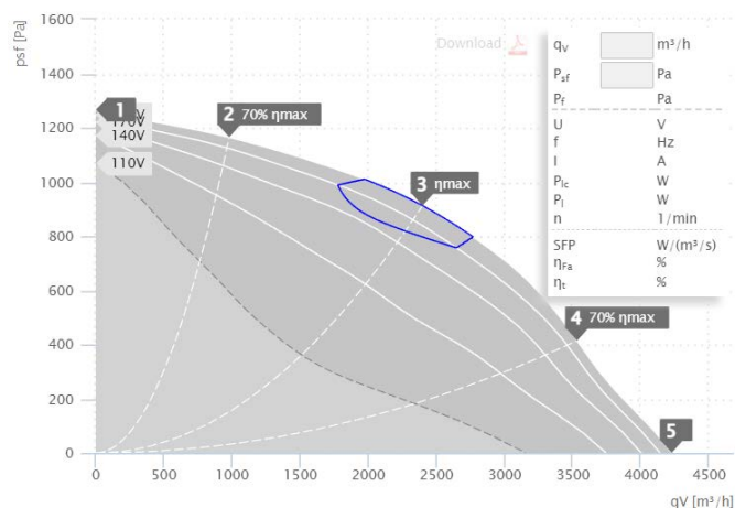
MPC 315 E2 T21 | 136829 (230V)
