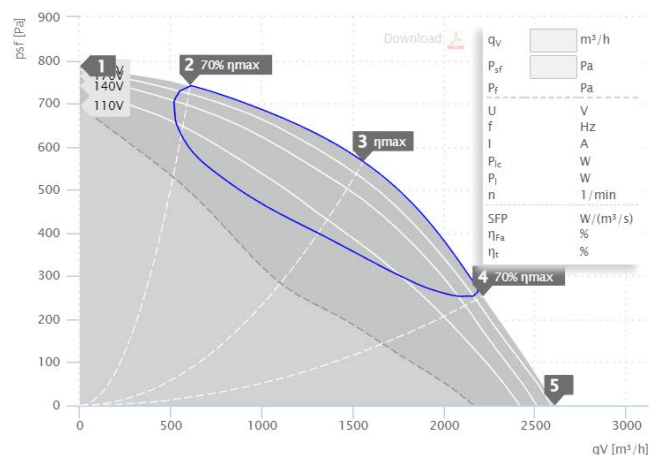
MPC 250 E2 T20 | 126679 (230V)
