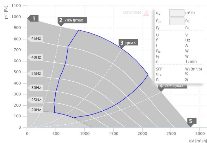
MPC 280 D2 T40 | 157214 (400V)
